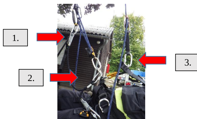
9. ábra Ereszkedőgép, mászógép, karabinerek összeállítása egy rendszerbe, mászás-ereszkedés biztonságos végrehajtásához, önbiztosítás alkalmazásával. Magyarázó ábra segítheti az eszközök biztonságos együtthasználtságának megértését (1=mászógép, 2=ereszkedőgép, 3=karabiner; Fotó: HUNOR Mentőszervezet)
